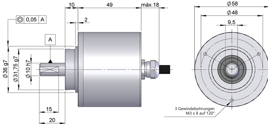
Maßzeichnung Vollwelle Typ 1, Anschluss 8, ohne Flansch
