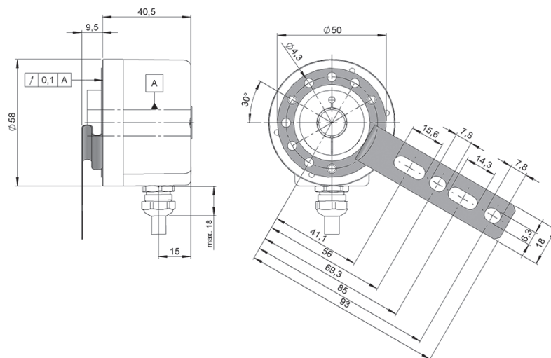
Flexible flange 90.1095
